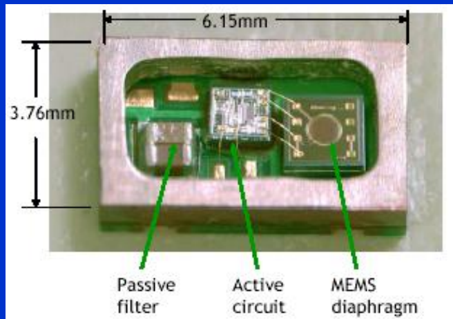
MEMS mikrofon
