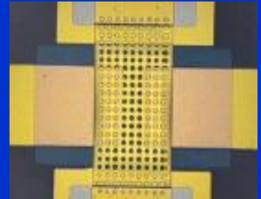
Mikrotalasni prekidač
