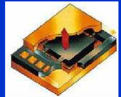
Senzor ubrzanja
